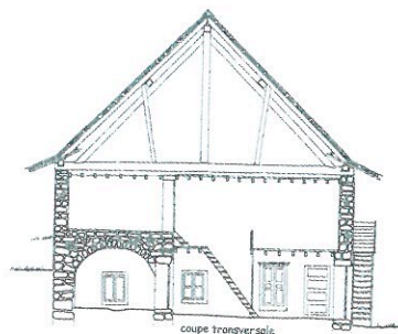
coupe transversale
