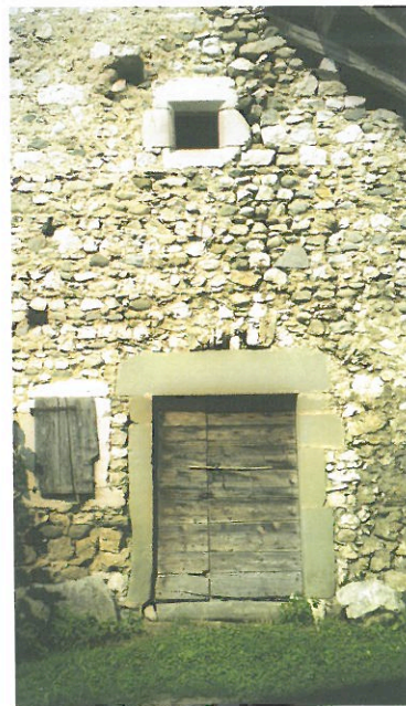
Les murs de cette grange sont constitués de moellons irréguliers. Les ouvertures sont encadrées de pierres taillées (calcaire et grès argileux). (Le Bourget-du-Lac, Savoie.)
