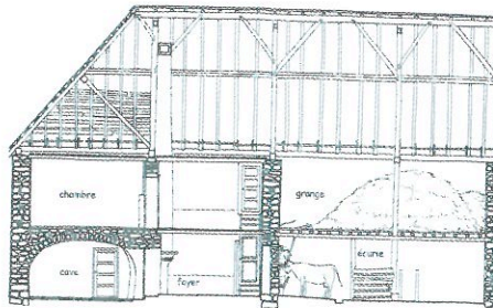
coupe longitudinale
