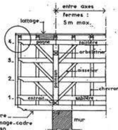
COUPE LONGITUDINALE
