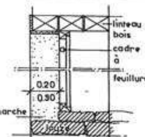
COUPE verticale
